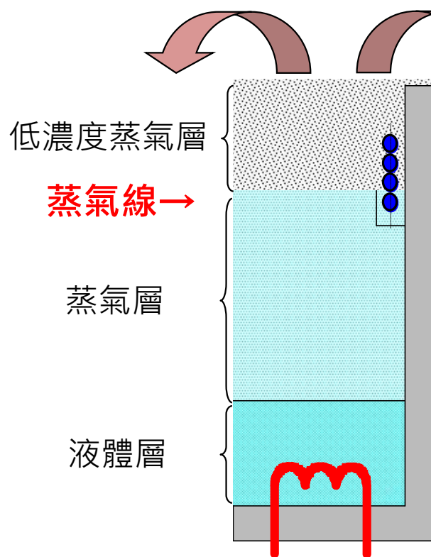
洗淨槽內示意圖
