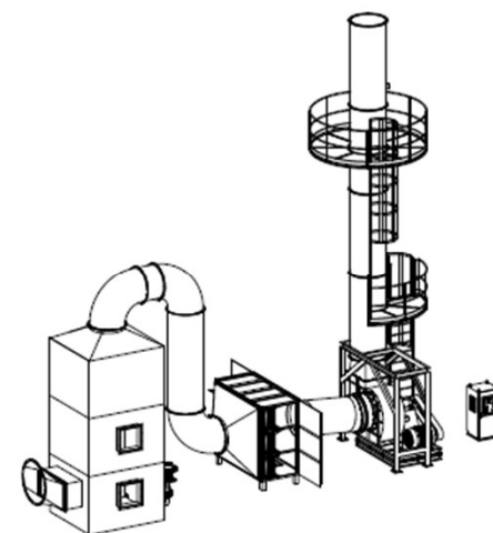
機組設備立體配置示意圖
